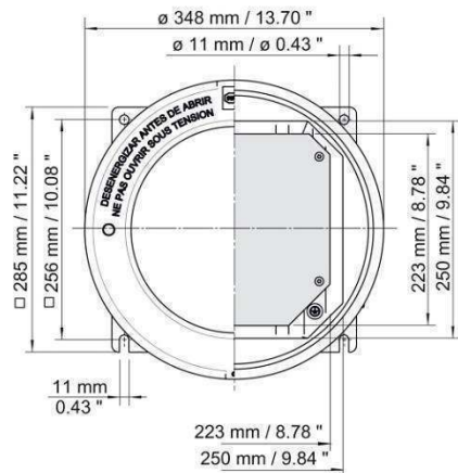
Gehäuse Größe 5 8265/5-000, ohne Schauglas
