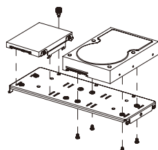
1 x 2.5" ; 1 x 3.5" HDD
