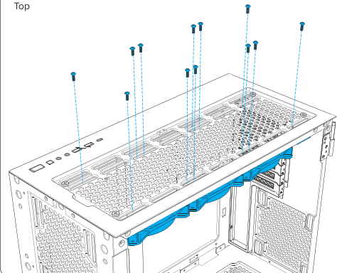
Top
