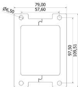
LGA 4189
