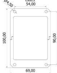
LGA 4189
