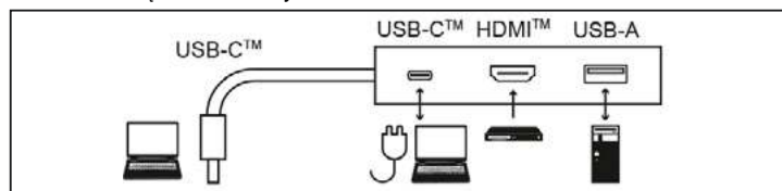
Fig.: Przyłącze
