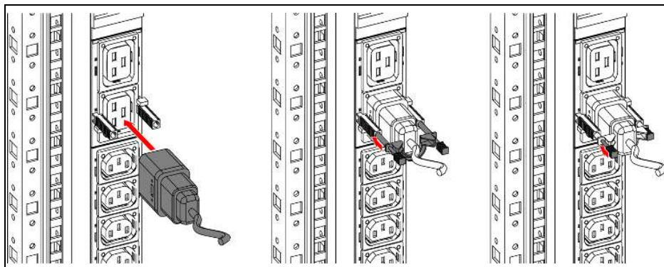
Abb./Fig./Fig. 11: Kabelbefestigung / Cable attachment / Blocage des câbles
