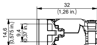
Einbaumaße / mounting dimensions
